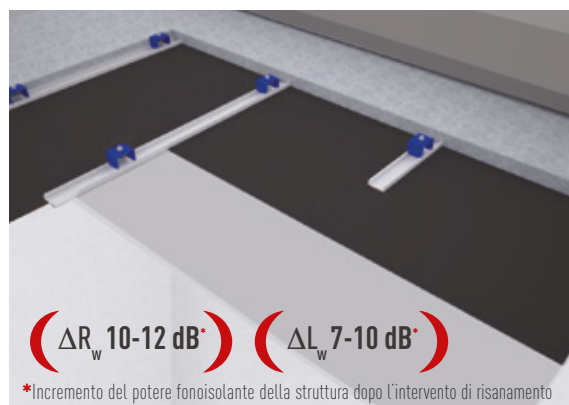
↑ Controsoffitto a basso spessore e finitura a singola lastra con IsolGypsum Telogomma o IsolGypsum Perfetto 10 mm avvitabile
